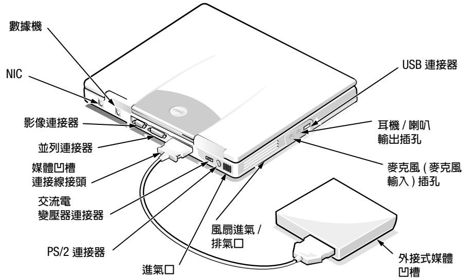
圖 3-5：電腦後視圖
